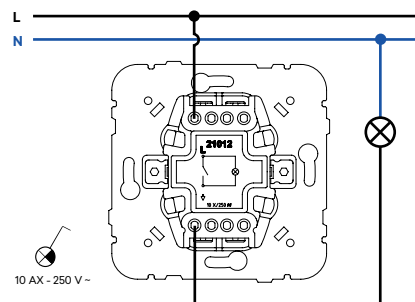
Interrupor Luminoso
