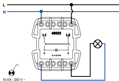
Interrupor Bipolar con Piloto de Señalización
