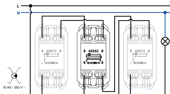
Conmutador de Cruce Luminoso
