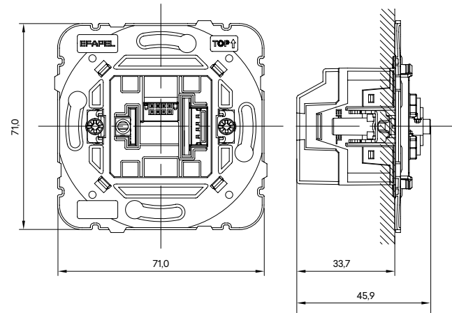
Dimensiones MEC 21 (mm)
