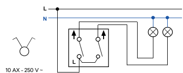
Doble Interruptor
