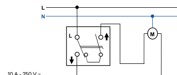
Interruptor para Persiana
