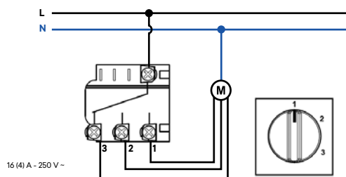
Interruptor Rotativo 3 Posiciones
