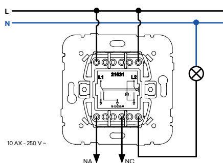
Interrupor para Tarjeta Card-system
