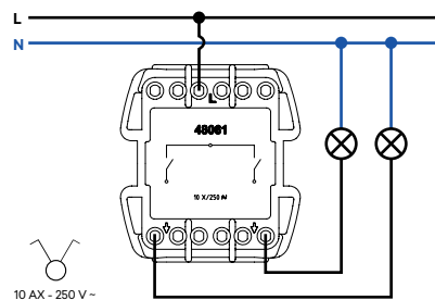
Doble Interrupor
