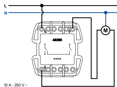
Interrupor para Persiana
