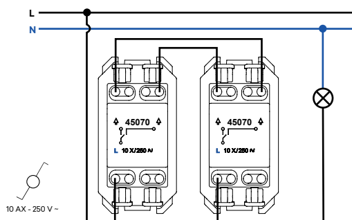
Conmutador
