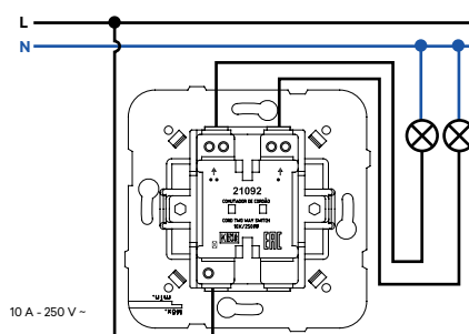
Conmutador con Tirador
