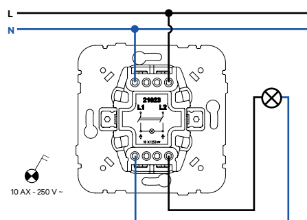
Interrupor Bipolar con Piloto de Señalización
