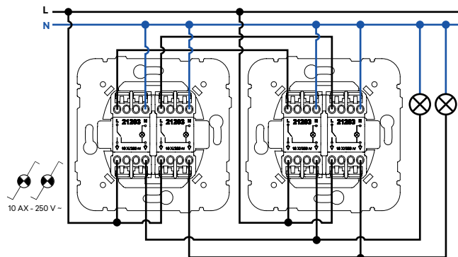
Doble Conmutador con Piloto de Señalización
