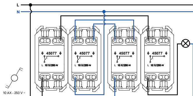
Conmutador Bipolar
