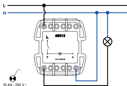
Interrupor con Piloto de Señalización
