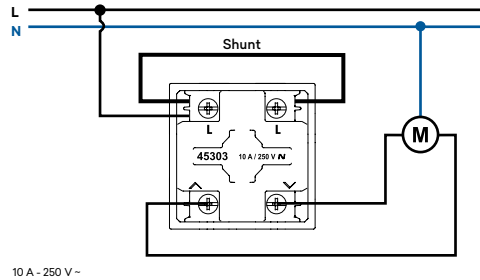
Pulsador Rotativo para Persianas
