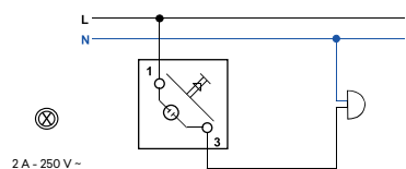
Pulsador Luminoso de 250 V ~
