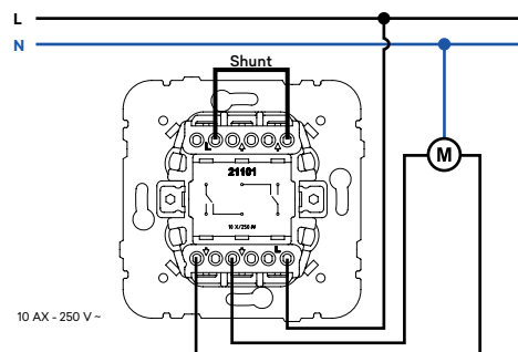
Mando Ventilador ON/OFF - 2 Velocidades
