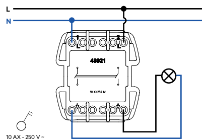
Interrupor Bipolar
