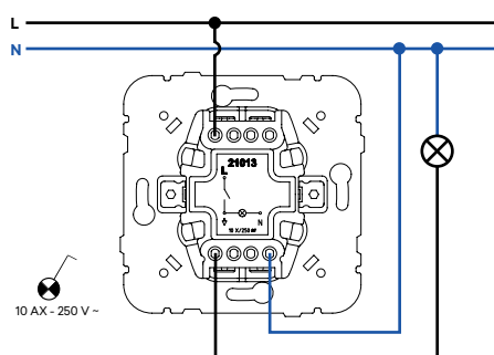
Interrupor con Piloto de Señalización
