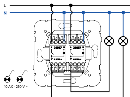
Doble Interruptor con Piloto de Señalización
