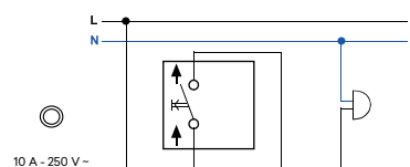
Pulsador
