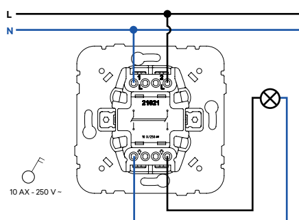
Interrupor Bipolar
