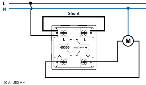
Conmutador Rotativo de Persianas
