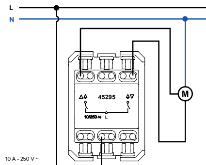
Interrupor para Persiana con Enclavamiento Mecánico
