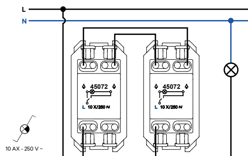
Conmutador Luminoso
