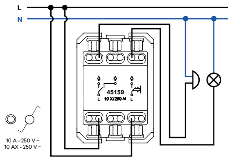
Pulsador / Conmutador
