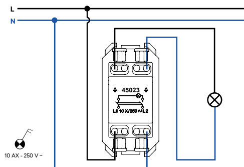
Interruptor Bipolar con Piloto de Señalización
