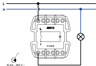
Interrupor Luminoso
