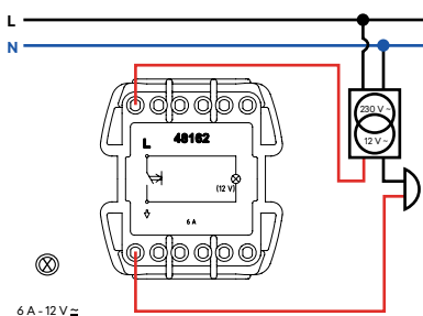
Pulsador Luminoso de 12 V =
