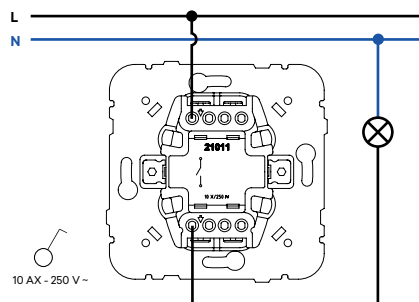
Interrupor Unipolar
