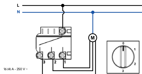
Interruptor Rotativo 4 Posiciones
