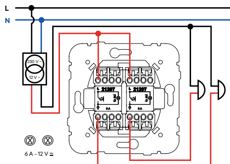
Doble Pulsador Luminoso 12 V ≈
