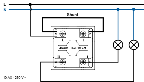
Conmutador Rotativo
