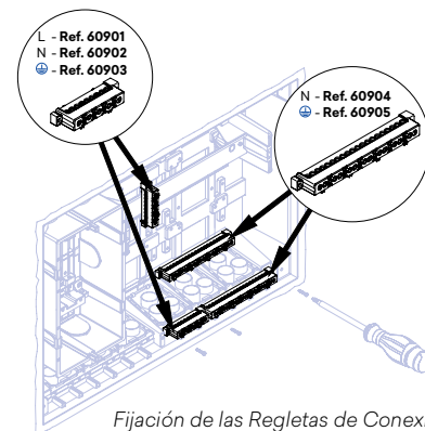
Fijación de las Regletas de Conexión
