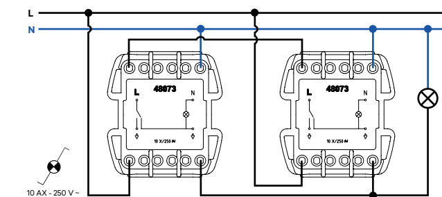
Conmutador con Piloto de Señalización
