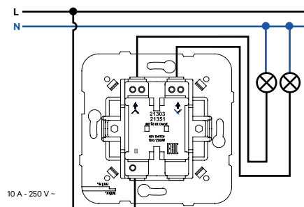
Pulsador Rotativo para Persiana | Pulsador con Llave
