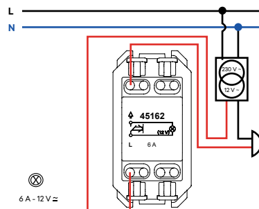
Pulsador Luminoso de 12 V ~
