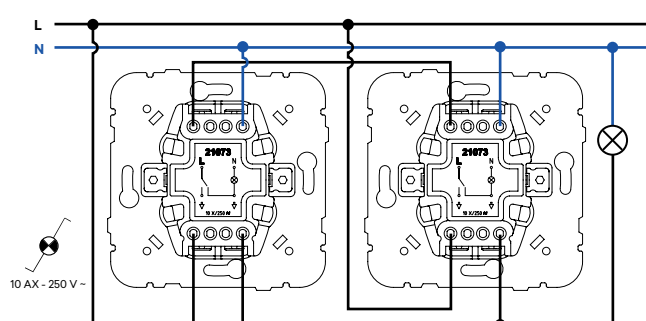
Conmutador con Piloto de Señalización
