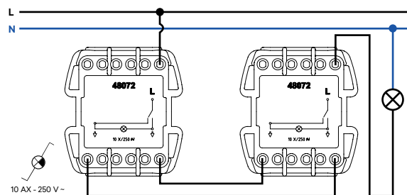
Conmutador Luminoso
